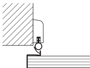
Боковой уплотнитель на вспомогательной замыкающей кромке
