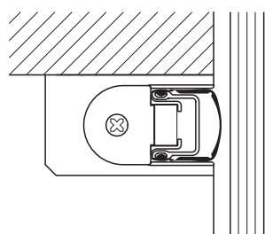
Дверной уплотнитель сверху на верхней кромке дверной коробки
