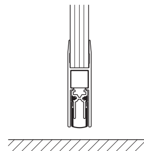
Дверной уплотнитель снизу на дверном полотне
