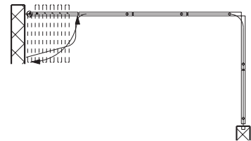
90°-Stapelung bei Anlage mit Richtungsänderung und Drehtüre.
